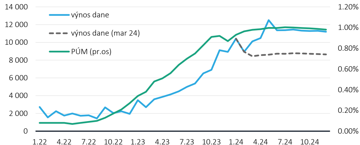
Mesačný vývoj úrokovej miery a výnosu dane
